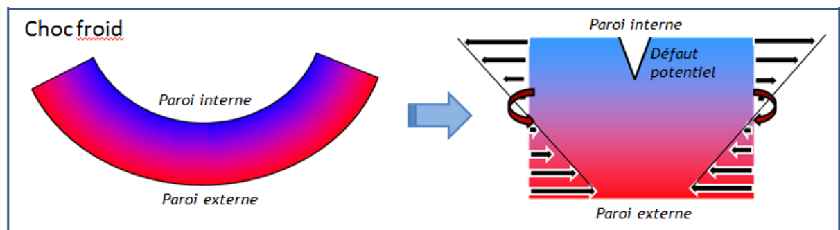
Répartition de la température dans la paroi du fond de la cuve de l'EPR en cas de choc froid ainsi que la répartition des efforts induits dans la paroi.
