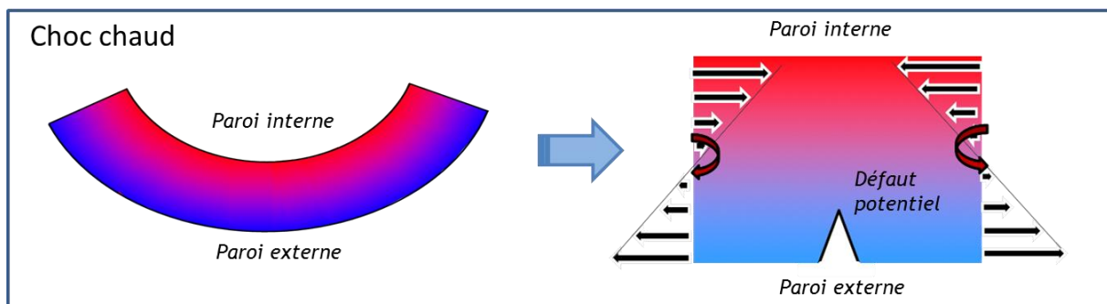
Répartition de la température dans la paroi du fond de la cuve en cas de choc chaud, et répartition des efforts induits dans la paroi.
